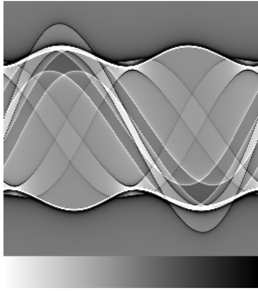
(c) フィルタ補正 q(X, \beta, Z = 0)
