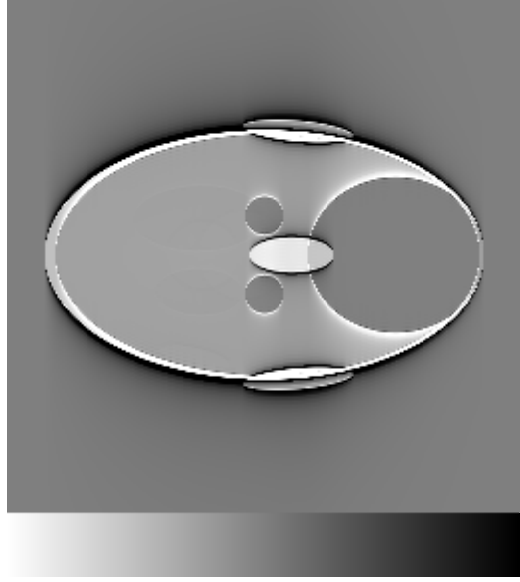
(b) フィルタ補正 q(X, Z, \beta = 0)
